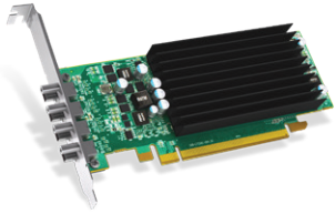
Matrox C420 P/N: C420-E4GBLAF
